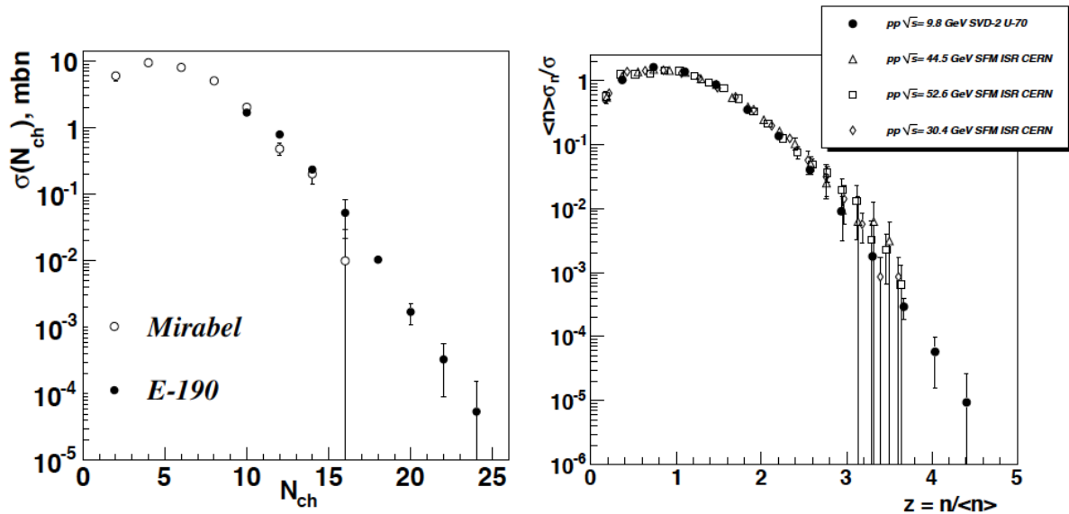
Рис. 2.(Слева) Топологические сечения, измеренные на установках Mirabelle (пустые кружки) и СВД-2 (сплошные кружки) при энергии протонного пучка 50 ГэВ.
