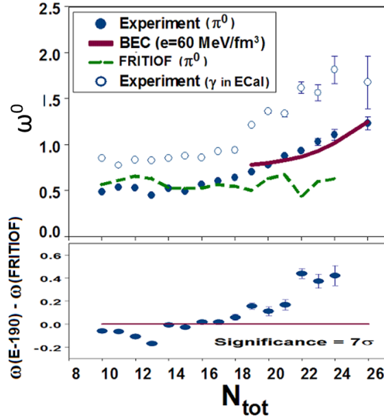
Рис. 8. Нормированная дисперсия, измеренная для \pi^0 (полные кружки) и \gamma (пустые кружки); теоретическое предсказание (коричневая линия) и результат Монте-Карло моделирования (зеленая линия).
