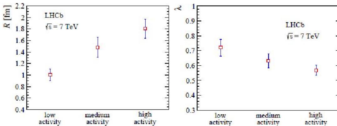
Рис. 9. Корреляционный радиус R и параметр хаотичности \lambda как функции активности [21].
