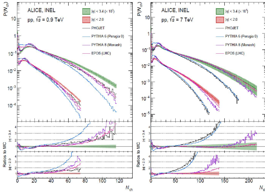
Рис. 1. Сравнение распределений по множественности для неупругих событий (Сотрудничество ALICE) с Монте-Карло генераторами PYTHIA 6, Perugia 0, PYTHIA 8 Monash, PHOJET и EPOS LHC при 0.9 (слева) и 7 ТэВ (справа). Объединённые статистические и систематические ошибки показаны полосами.
