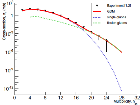
Рис. 4.(Слева) Описание данных СВД-2 моделью МГД с учетом ветвления глюонов. Синяя штриховая линия соответствует вкладу от адронизации одиночных глюонов, зелёная – от адронизации двух глюонов, один из которых появляется за счет деления.
