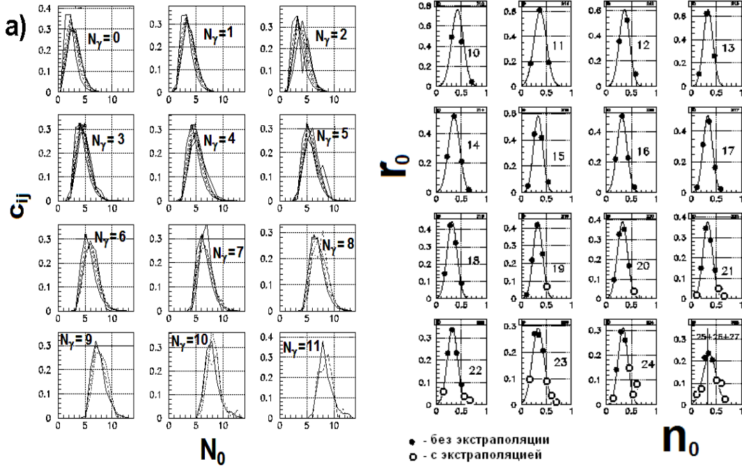
Рис. 6.(Слева) Весовые коэффициенты c_{ij} [14-15].
